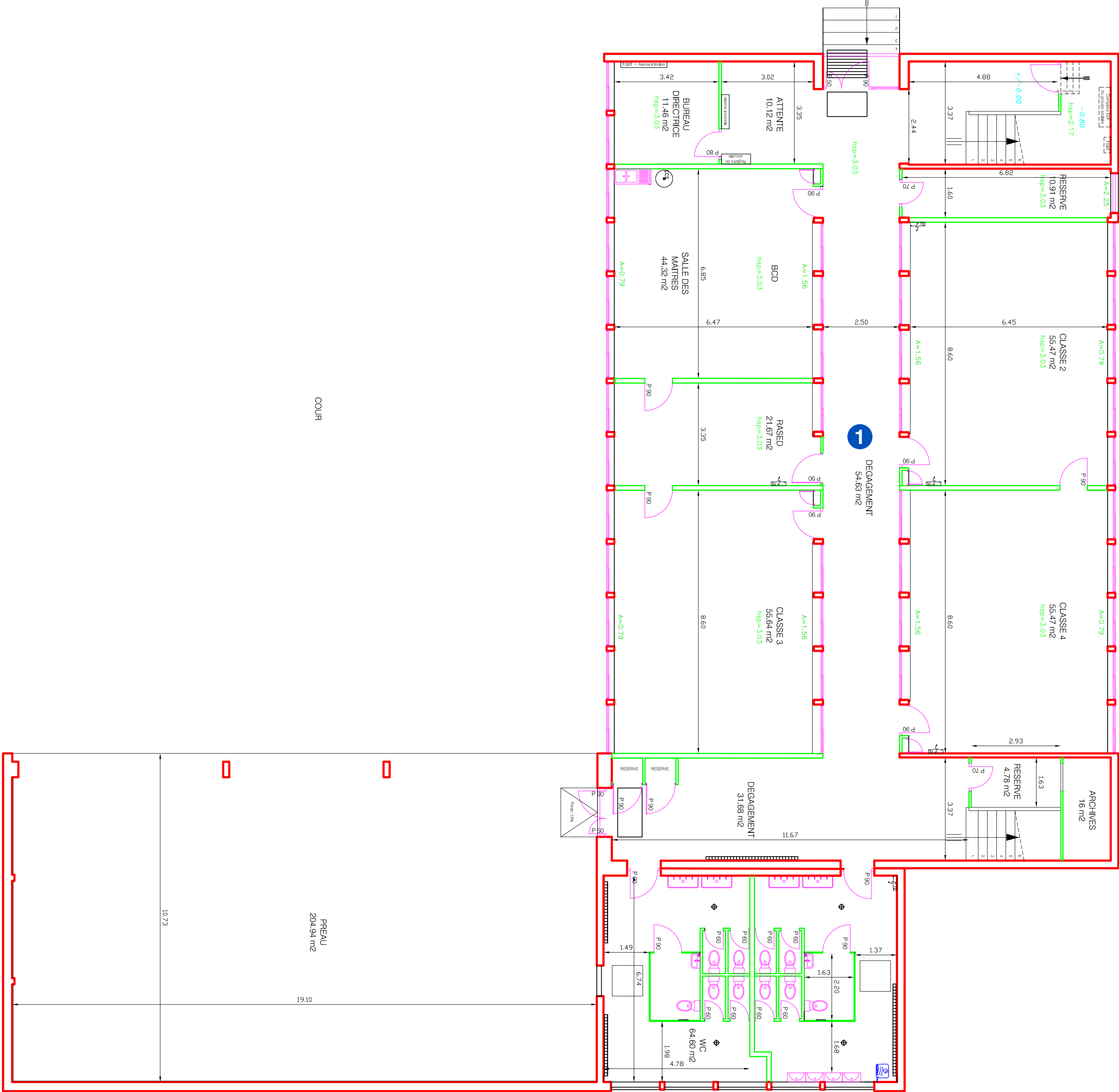
ECOLE ELEMENTAIRE - PAUL LANGEVIN 1 - RDC
